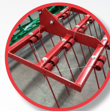
Rastras de púas de 2 o 3 filas. 2 or 3 rows tine harrow.
